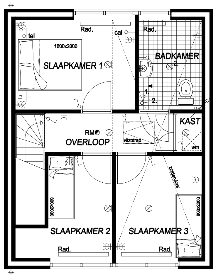
VERDIEPING
